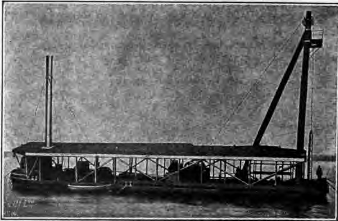
Fig. 179. A Lobnitz Rock Breaker.
